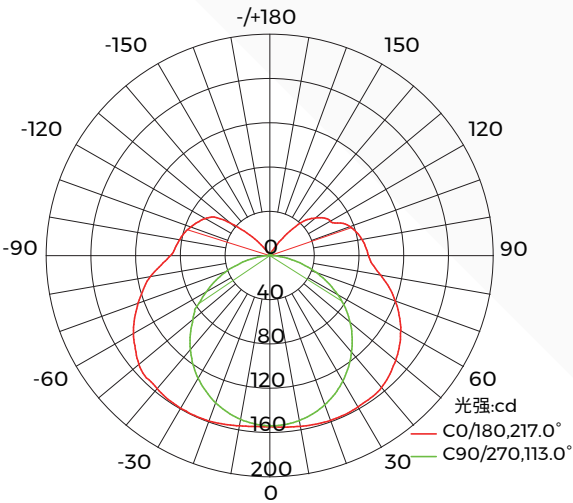
配光曲线
