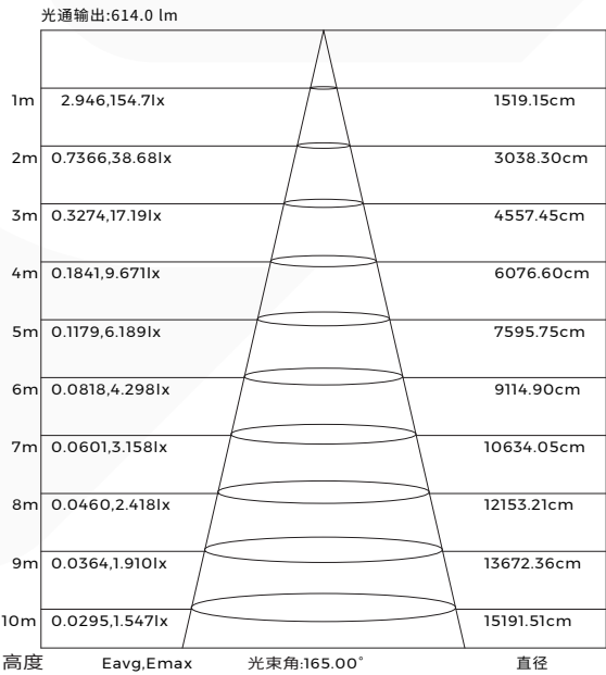
注:曲线为灯具在不同投射距离下的照射区域及区域内平均照度 有效平均照度
